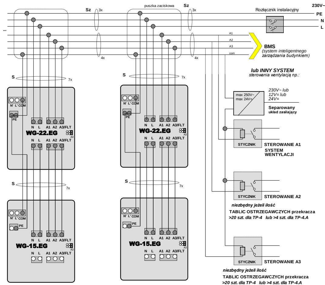
Rys.3. System 3-progowy (lub 2-progowy z sygnalizacją stanu AWARIA), obwody sterujące ODSEPAROWANE od zasilania – możliwość współpracy z BMS lub innymi systemami sterowania wentylacją
