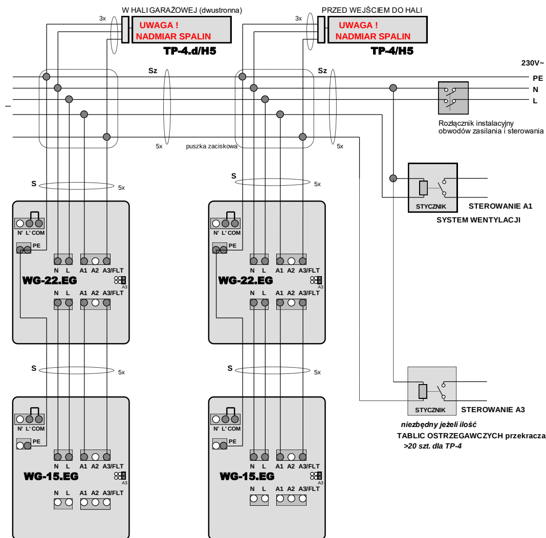
Rys.1. System 2-progowy, OPTYMALNY ekonomicznie , przewody sterujące zwierane w stanie alarmowym do przewodu fazowego (bez napięcia w czasie stanu normalnego);
