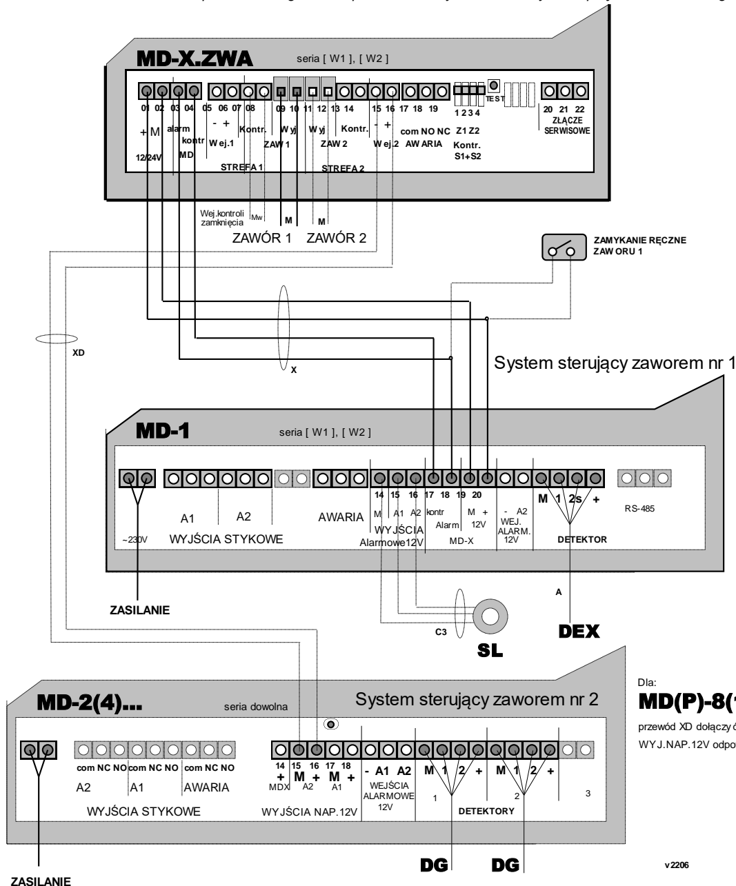
RYS.1.1. SCHEMAT BLOKOWY SYSTEMU
