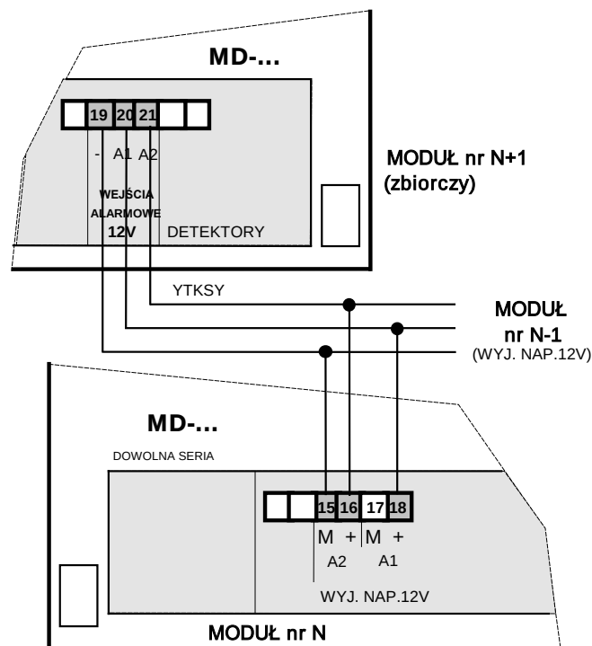
Kaskadowe łączenie modułów MD
