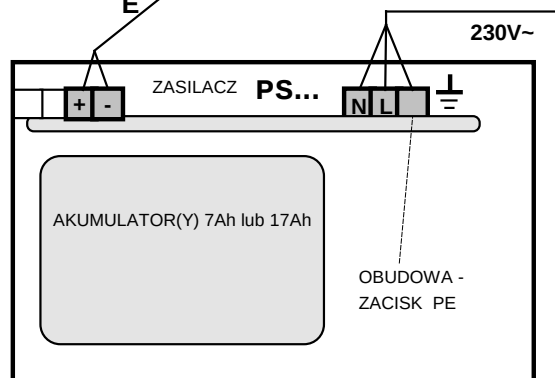
Podłączenie zasilania 12V=
