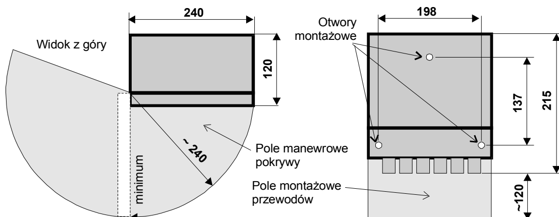
Rys.2. Wymagane pole montażowe.
