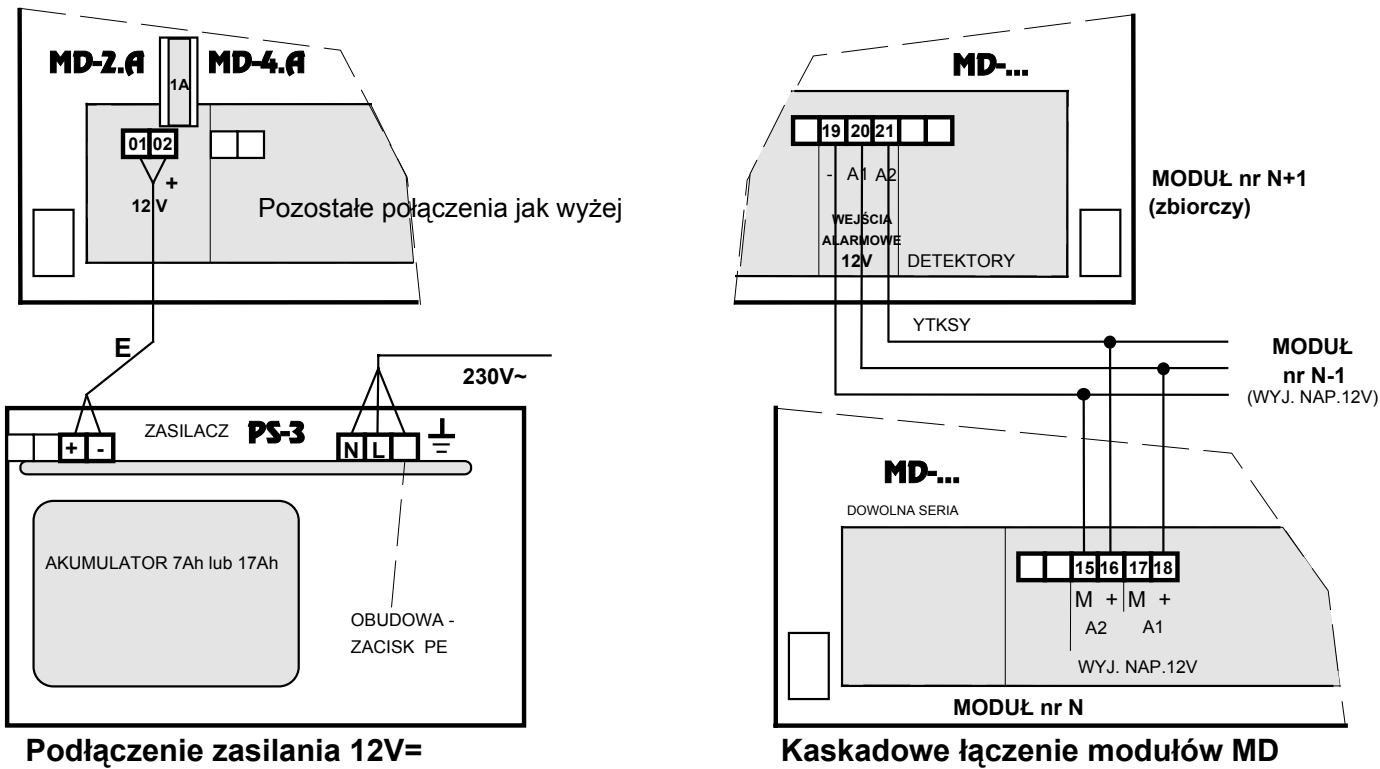
Rys. 3.2. Widok komory zaciskowej – połączenia elektryczne
