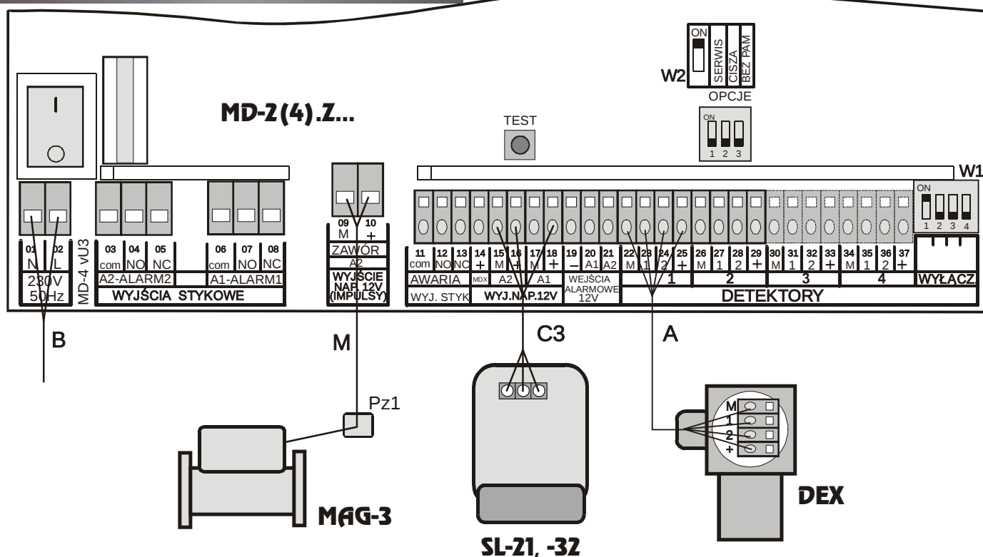
Rys.3.2 Widok komory zaciskowej modułu i podłączeń przewodowych
