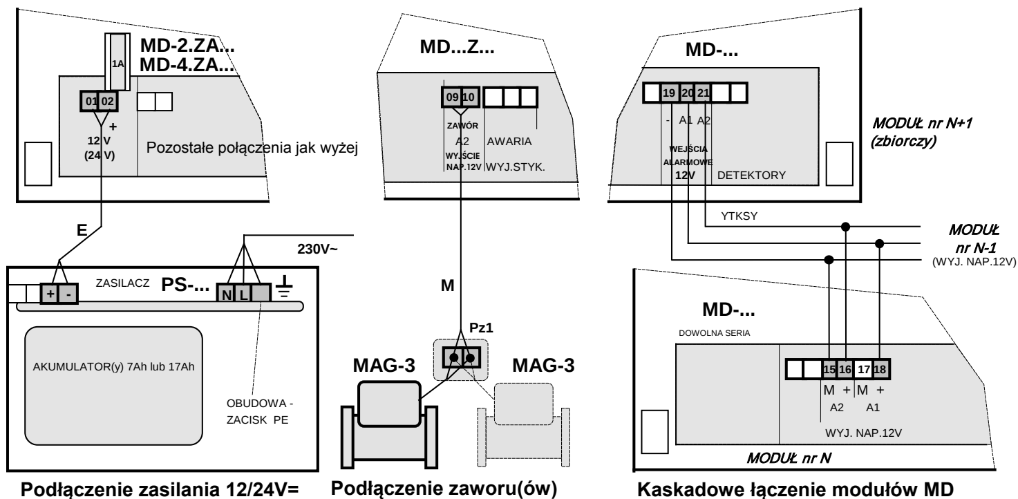
Rys.3.2.A Połączenia przewodowe różnych wariantów systemu
