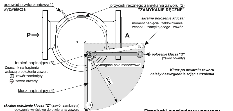
Przekrój poglądowy zaworu
