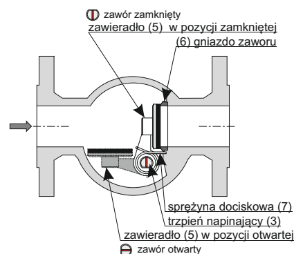
Przekrój poglądowy zaworu
