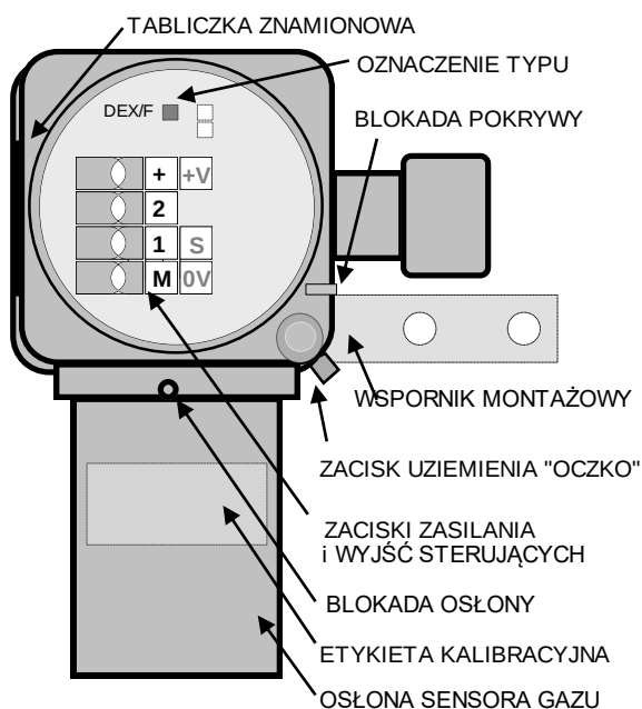
Rys.3.1. Widok bez pokrywy
