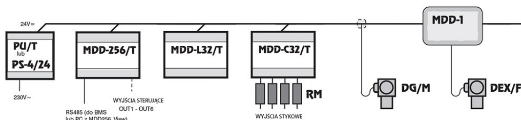
Schemat ideowy przykładowego, rozległego, Cyfrowego Systemu Detekcji Gazów
